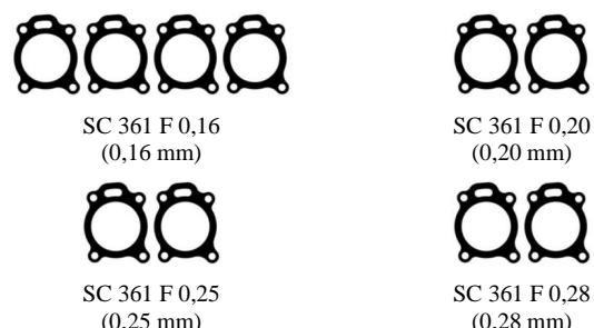
SCCA 06890 Jogo de calço da transferência para caixa de marchas
