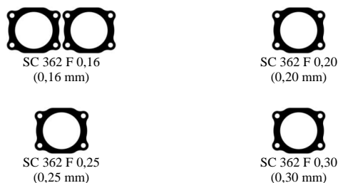
SCCA 06870 Jogo de calço de ajuste de pinhão
